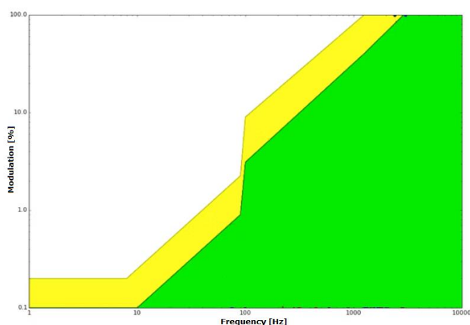
Figura 7: Soglia di percezione del Flickering
