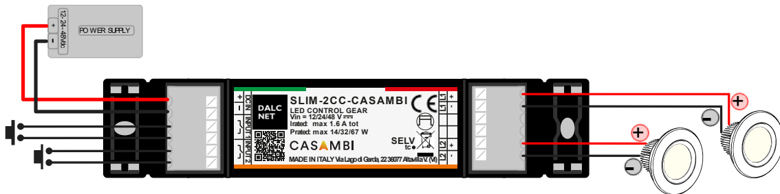
Figura 2: Schema di collegamento per carichi LED bianchi o monocolori
