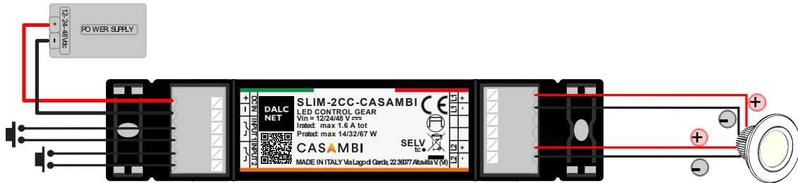
Figura 3: Schema di collegamento per carico LED Bianco Dinamico o Dim-to-Warm
