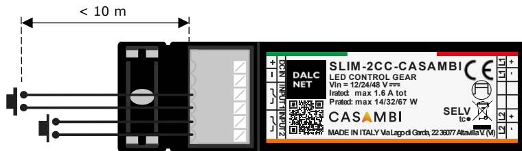
Figura 4: Schema di collegamento del comando locale per brevi distanze
