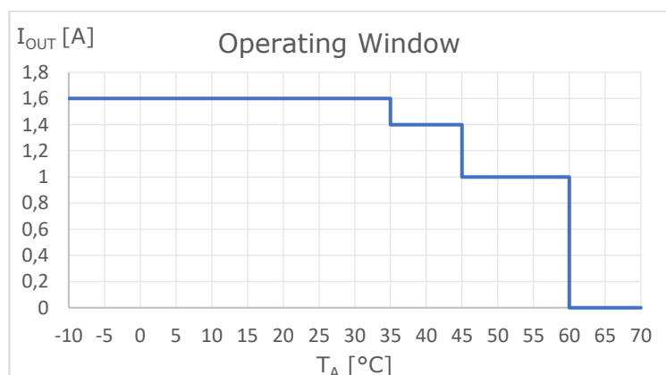
Figura 8: Finestra della temperatura di esercizio
