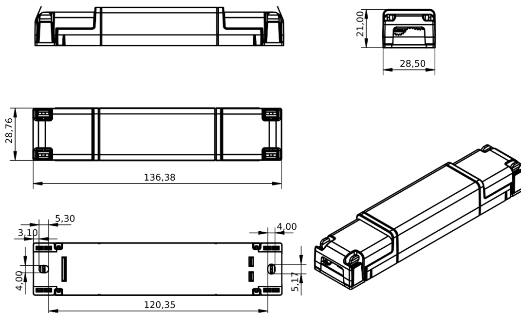
Figura 10: Dimensioni meccaniche
