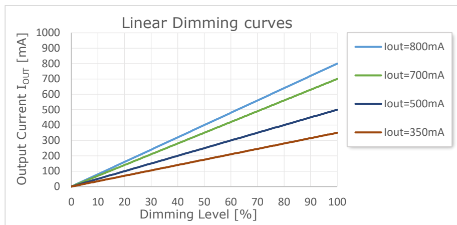
Figura 9: Curve lineari in base alla corrente di uscita impostata
